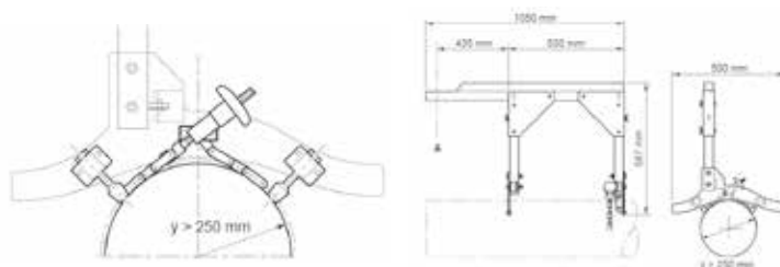
Support de tube petit diamètre
